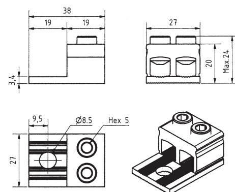
KKL 2x50
