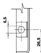
Detalle C
