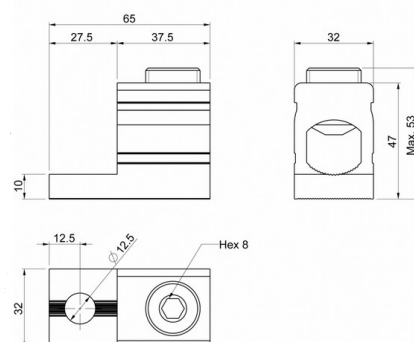
KKL 1x240
