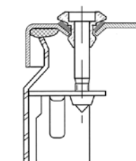
Detalle B
