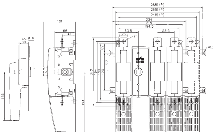
Cotas 315/400 A 3 y 4 polos
