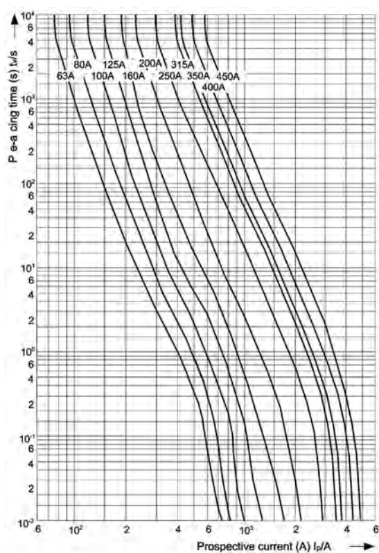
Gráfica curvas de disparo cartuchos NH1, 2 y 3 de 1100 V. M1DC, M2DC y M3DC
