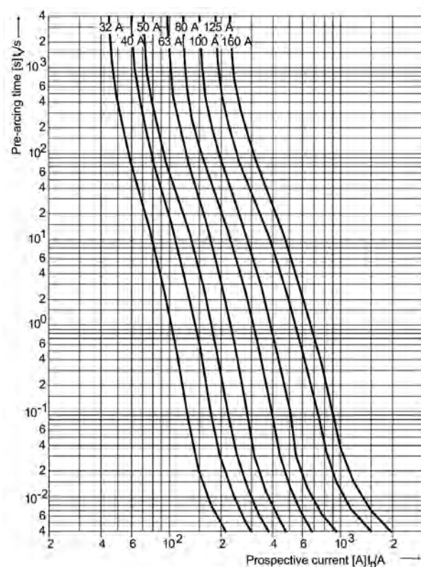
Gráfica curvas de disparo cartuchos NH1, M1DC... / 750 V
