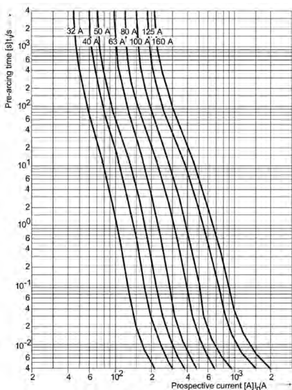
Gráfica curvas de disparo cartuchos NH1, M1DC... / 1000 V y MDC1... / 900 V
