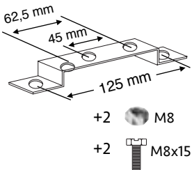
EM00420 bastidor metálico para SE00420 y SE00225
