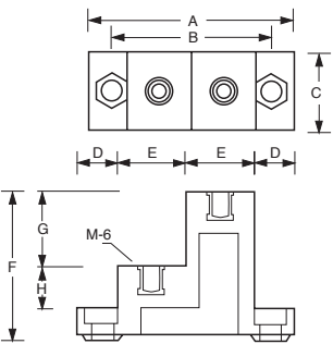
SE00215 pletinas hasta 15 x 5 mm
