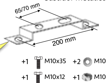
EM00430 bastidor metálico
